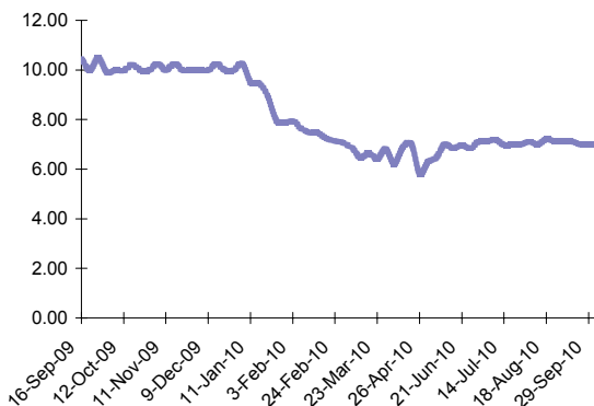
(%) Evoluția randamentelor 1 anualizate ale titlurilor de stat active în lei, perioada septembrie 2009- septembrie 2010
