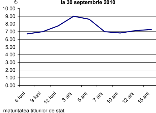
(%) Curba de randament 2 a titlurilor de stat în lei active la 30 septembrie 2010
