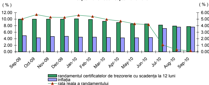
Inflația și randamentul certificatelor de trezorerie cu scadența la 12 luni septembrie 2009 - septembrie 2010
